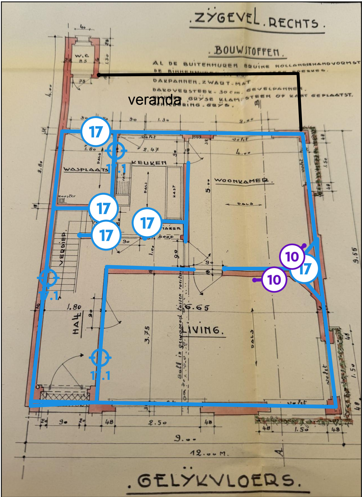
Legende van plan 1.4: Plan gelijkvloers
