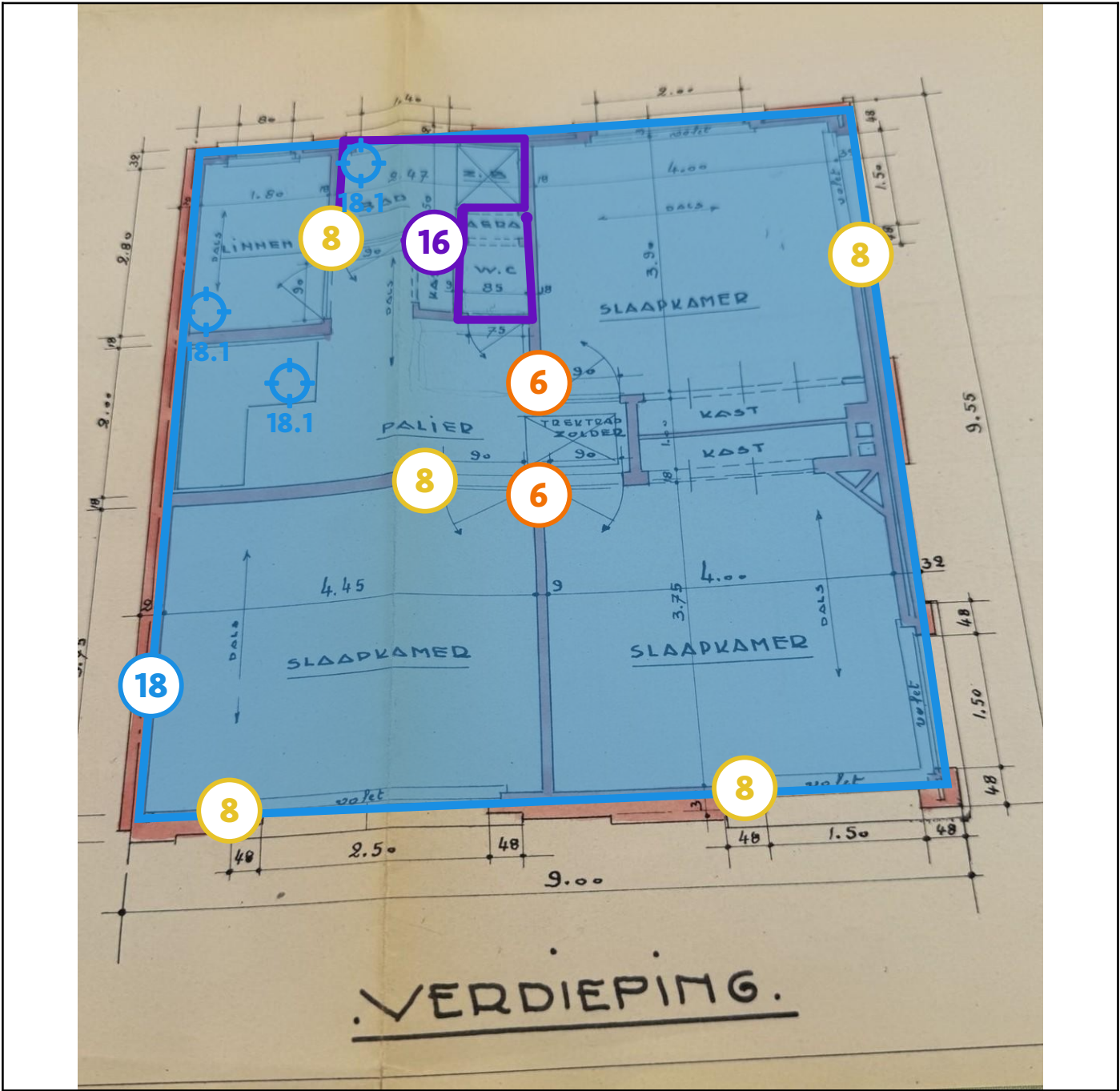
Legende van plan 1.5: Plan verdieping
